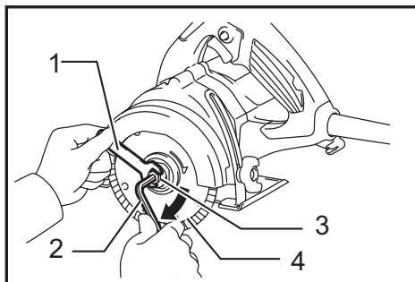
► 1. Clé 2. Clé hexagonale 3. Bague externe 4. Meule diamantée
