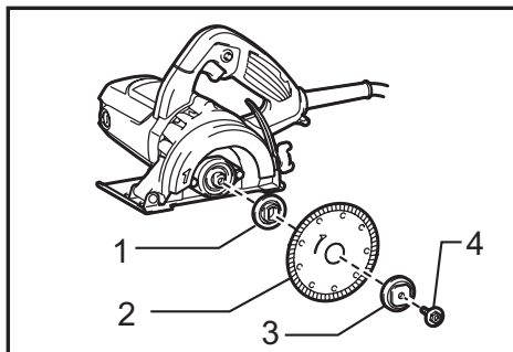
► 1. Bague interne 2. Meule diamantée 3. Bague externe 4. Boulon hexagonal
